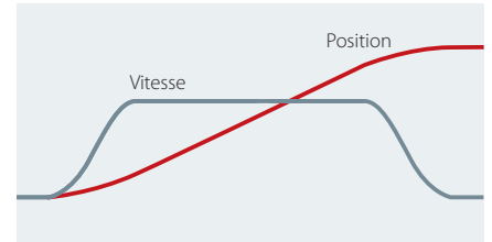
Fig. 2. Profil de mouvement avec rampes S
